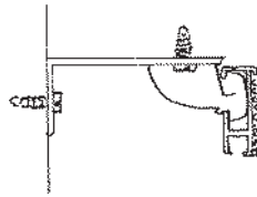
Tarrakiskon asennus kulmakannattimella seinään
