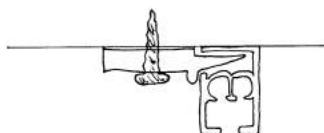
Kisko kattokannakkeessa
